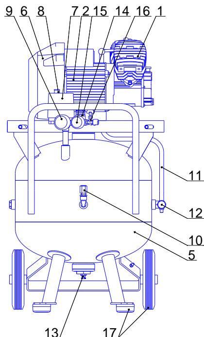
Рисунок 10 - Общий вид компрессора СБ4/С-50.J2047BV
