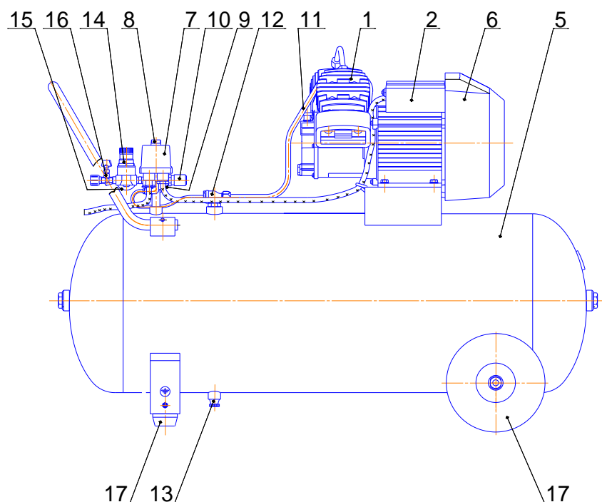
Рисунок 9 - Общий вид компрессора СБ4/С-100.J2047В
